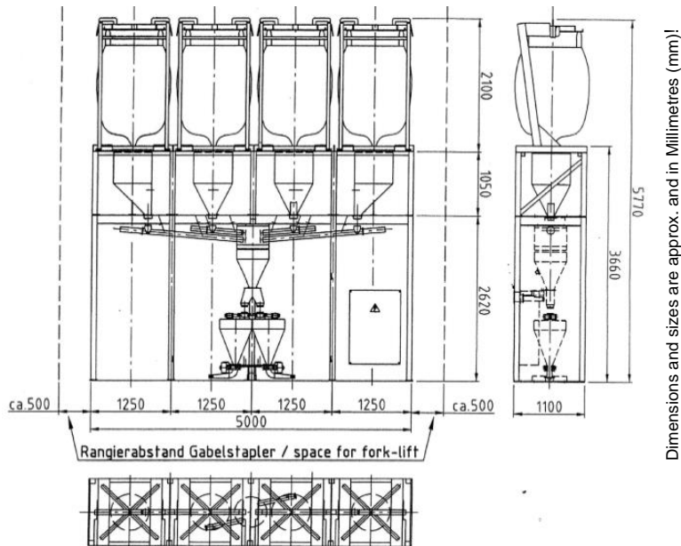
Dimensions FD 4 DS (double feeder)
