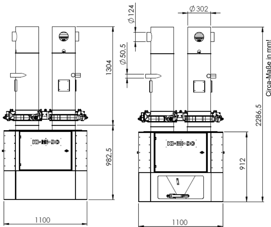
Abb. Maße PDE 75/4 – für 1 – 4 Komponenten
