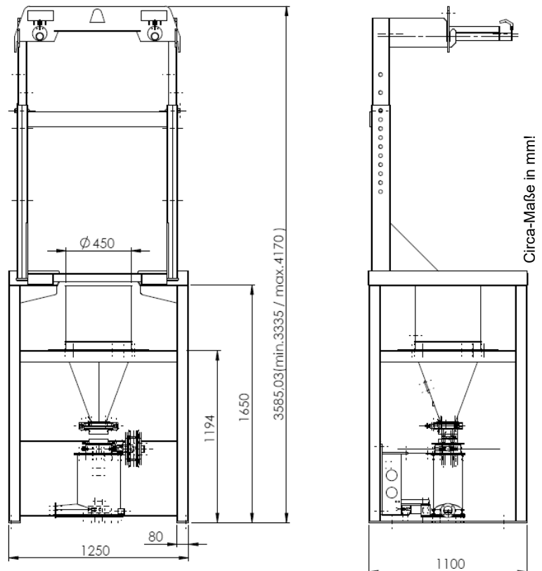
Abb. Maße Big-Bag-Förderstation BF 1500 für 1 Komponente
