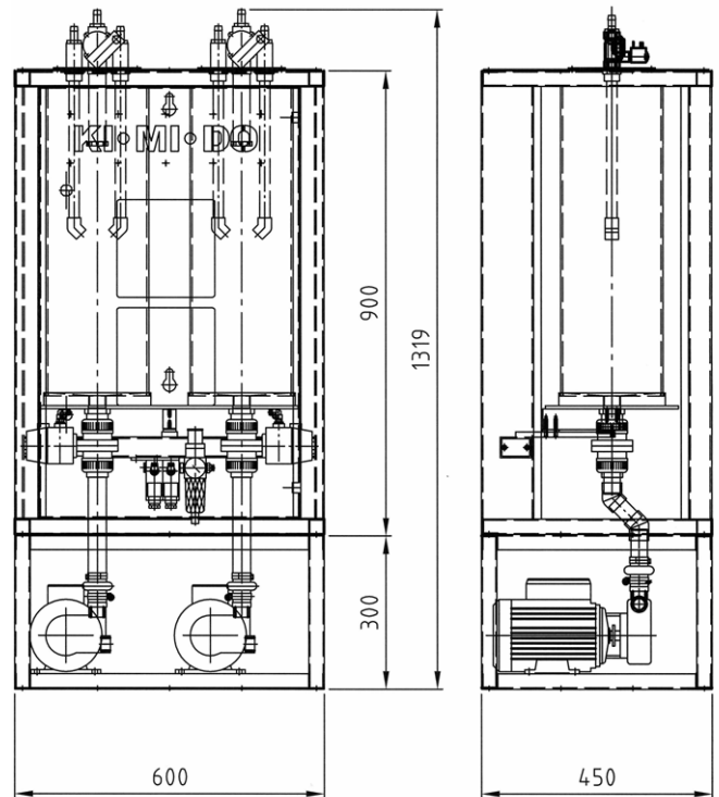
Schrankwaage SBW II 15/15 (Grundmodell) Innenansicht
