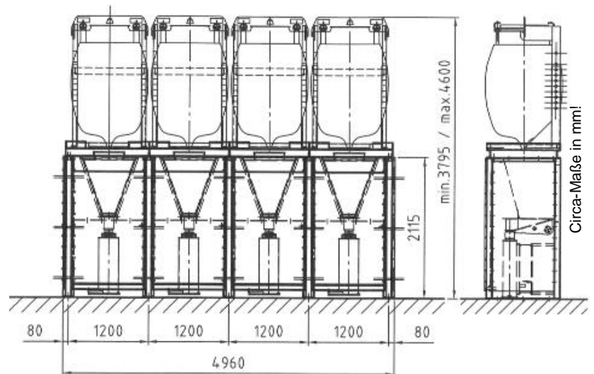
Abb. Maße PFD 4 WS
