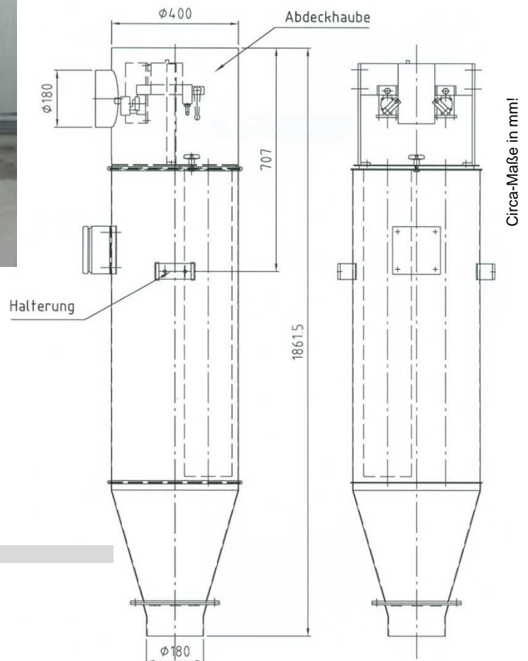
Abb.: Maße Mischersaugentlüftung Gr. VII 7,5 m 2 gemäß Zeichnung 0200.0500.62
