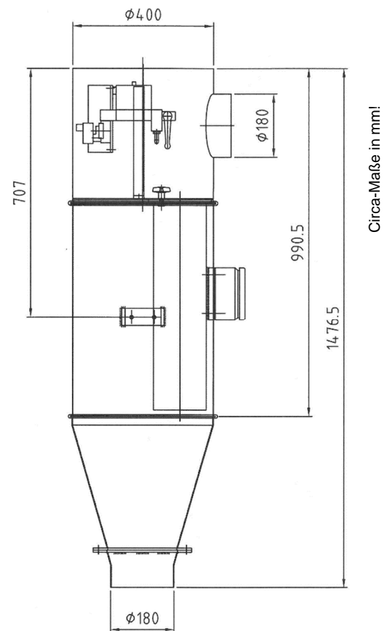
Abb.: Maße Mischersaugentlüftung Gr. V 4,5 m 2 gemäß Zeichnung 0200.0400.60
