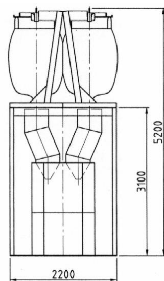
Maße MB 4 WS
