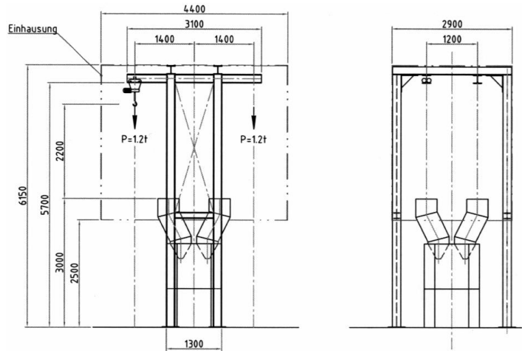
Maße MB 4 WS-K Kranbeschickung
