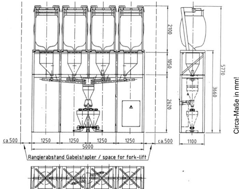
Abb.: Maße FD 4 DS (Doppelsender)
