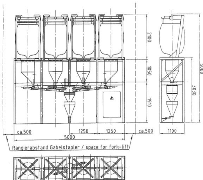
Maße FD 4 WS (Wägesender)
