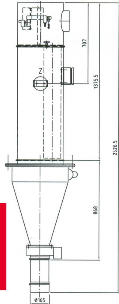
Fig. Dimensions size VII 7,5 m 2 , V= 60 l
