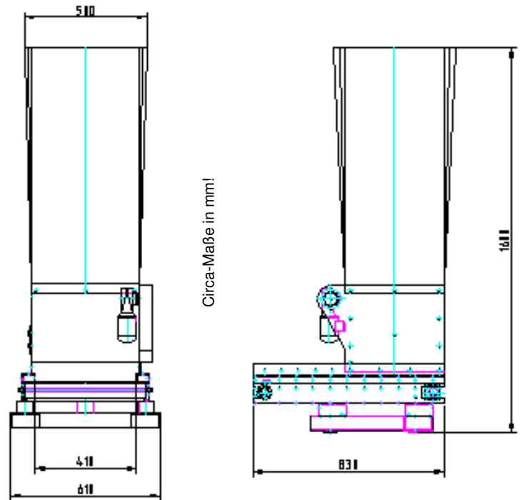
Abb.: Faserdosiergerät F-4R/400
