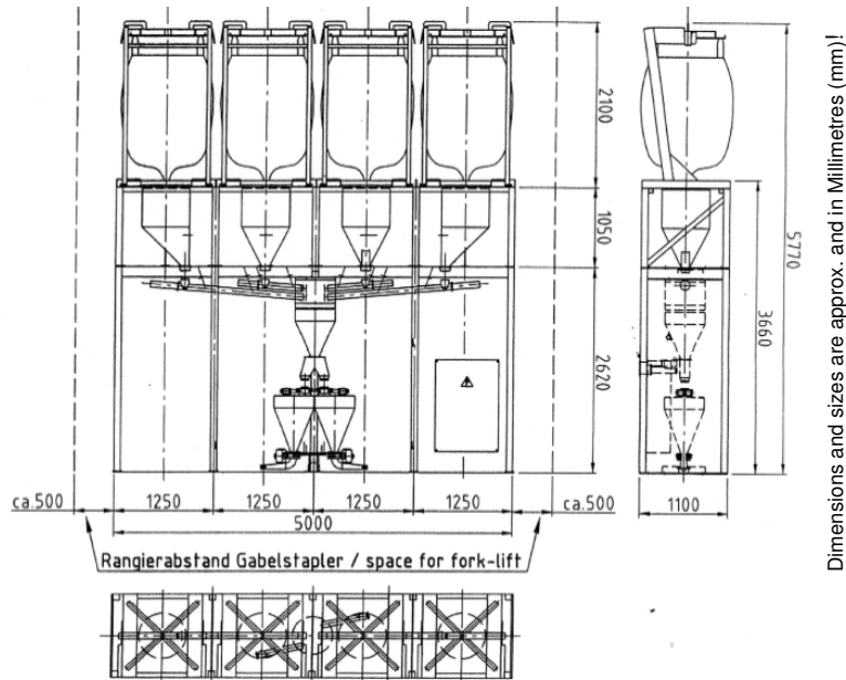
Fig.: Dimensions FD 4 DS (double feeder)
