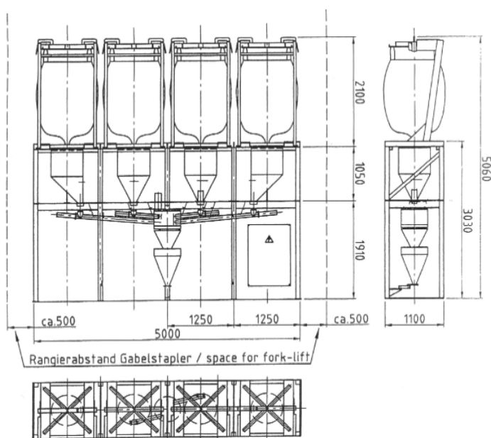
Abb.: Maße FD 4 WS (Wägesender)
